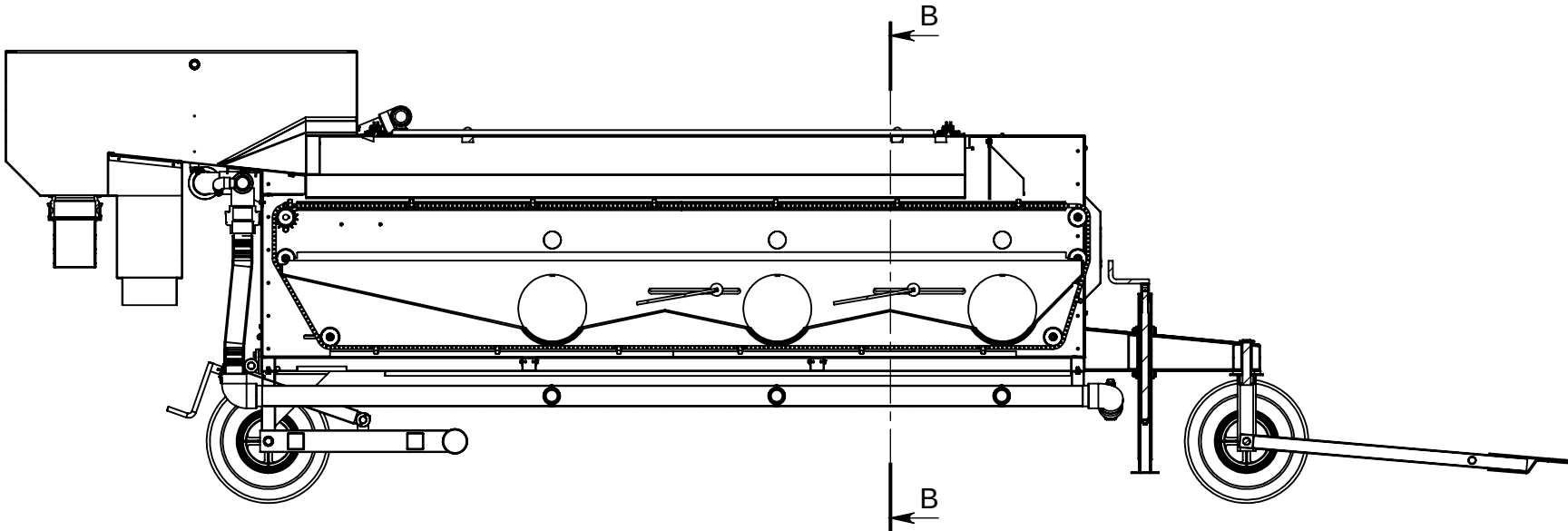
COUPE A-A
